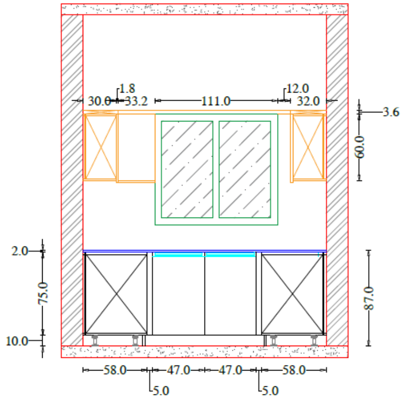
Elevation B
