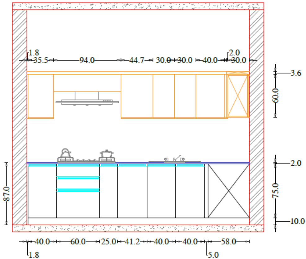
Elevation A
